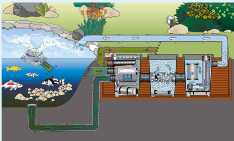
▲ Schematische Darstellung: Gravitationspumpe AquaMax Eco Gravity in Kombination mit den OASE Modulfiltren Proficlear Premium
