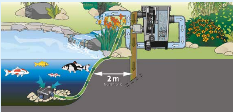
▲ Schematische Darstellung: ProfiClear Premium Compact gepumpt
