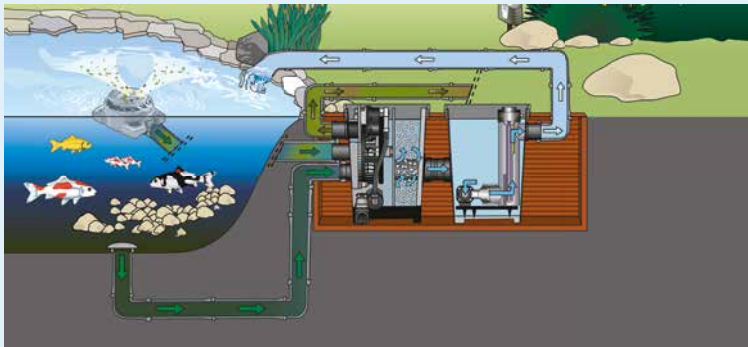
▲ Schematische Darstellung: ProfiClear Premium Compact Gravitation
